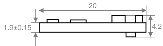
EDC158S-B (排针焊接孔: \phi 1.0\text{mm} ) 单位: (mm)
