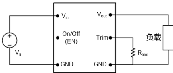
图 5-5 R trim 外部连接
