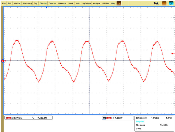
输出电压纹波 (对于图4-2B和C点, V_{in}=5V , V_{out}=1.2V , I_{out}=6A )
