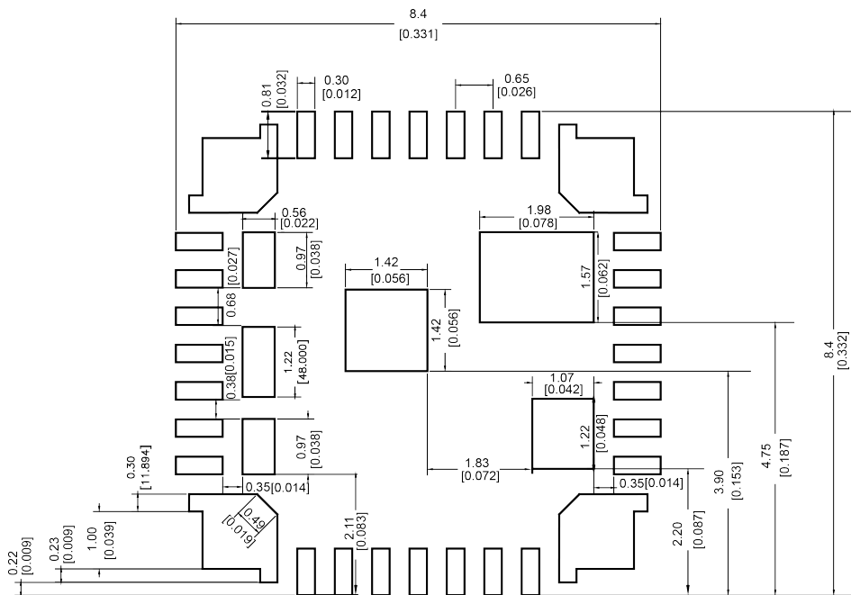
图 5-1 封装尺寸图
