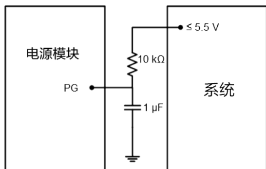
图 5-6 PG 配置图
