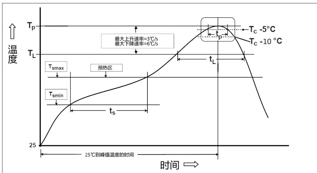
图 9-2 推荐无铅焊料回流曲线
