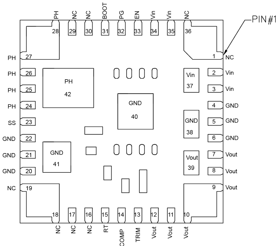
图 5-3 引脚分布
