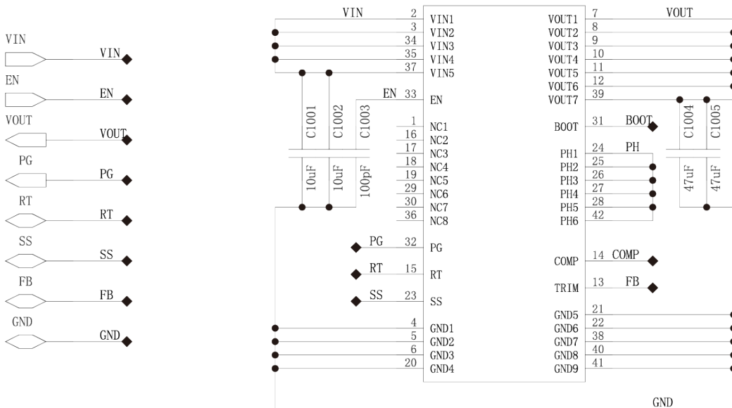
图 4-1 推荐应用电路
