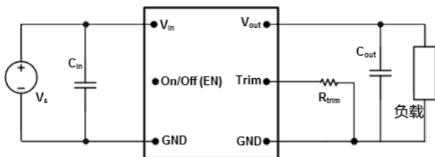
图 4-3 应用电路图
