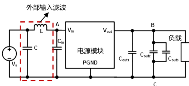
图 4-2 测试电路图
