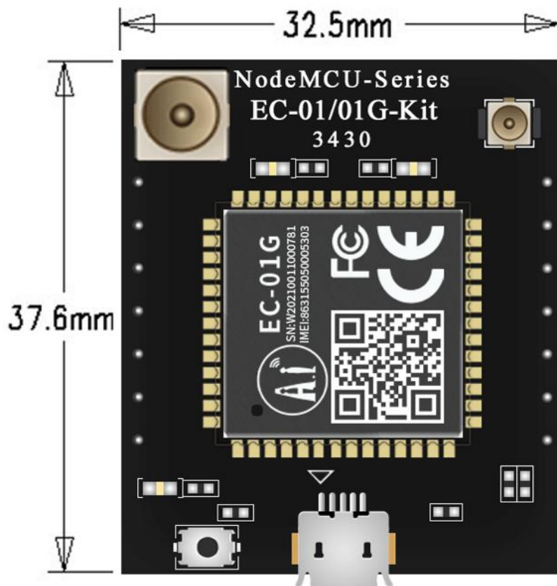
图 5 开发板尺寸图
