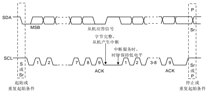
图 21 I 2 C 总线应答位
