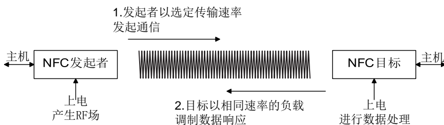
图 10 被动通信模式
