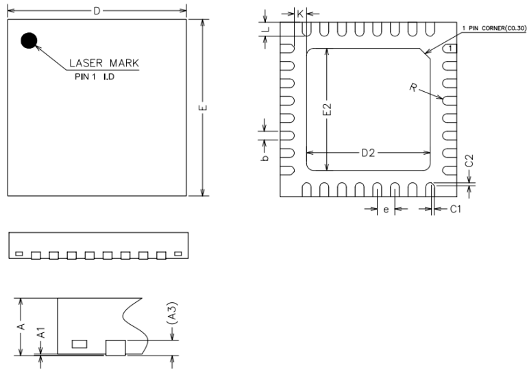
图 39 Si512 封装示意图
