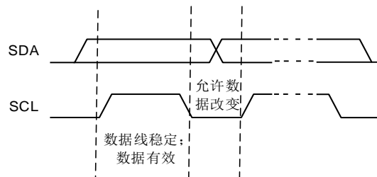
图 19 I 2 C 总线比特传输
