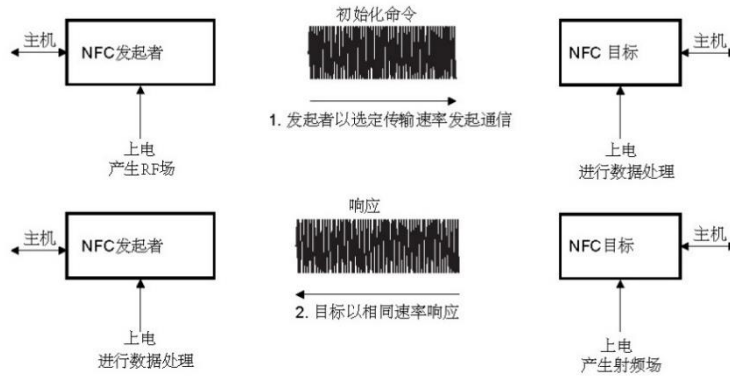
图 9 主动通信模式
