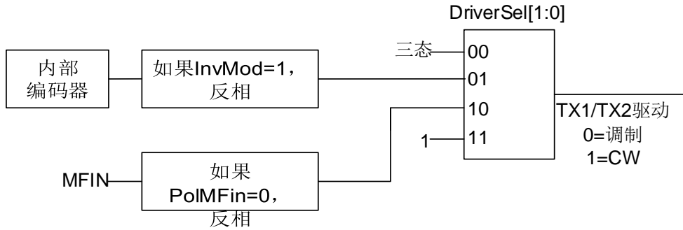
图 28 TX1 和 TX2 串行数据转换
