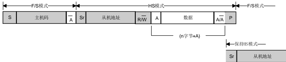
图 25 I 2 C 总线 HS 模式协议转换
