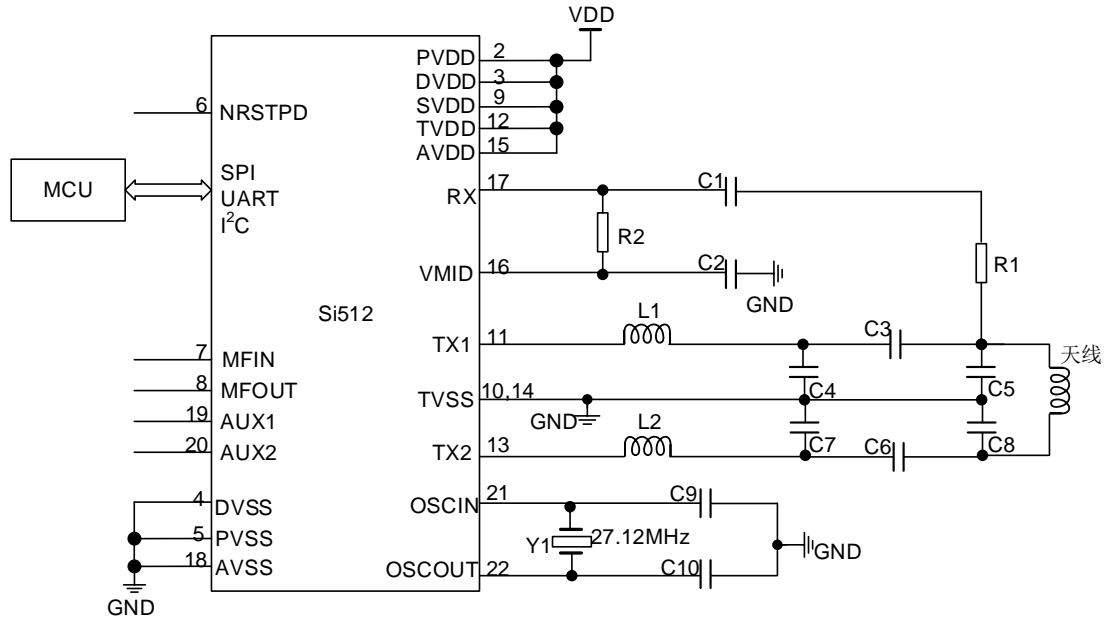
图 37 Si512 典型应用电路图-1
