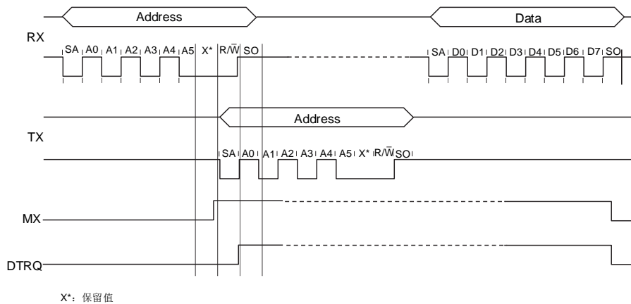
图 17 UART 写数据时序图
