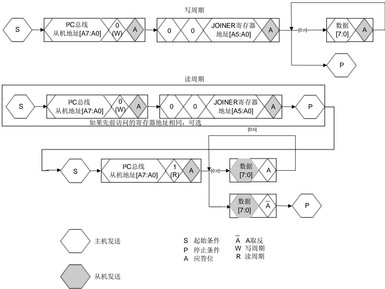
图 24 寄存器读写访问
