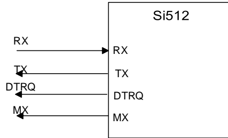
图 15 UART 接口
