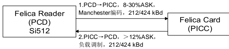
图 7 Felica 读卡器模式通信示意图
