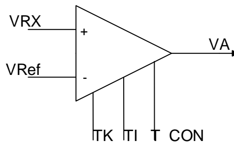
图 13 检波电路框图
