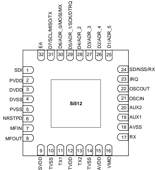
图 3 Si512 管脚示意图
