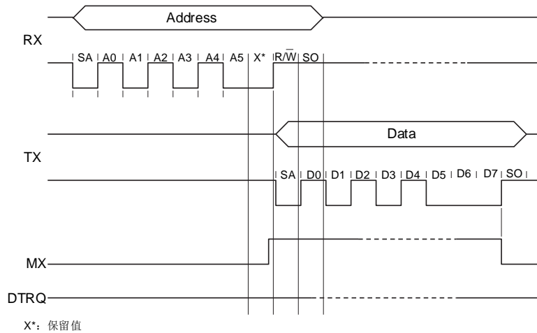
图 16 UART 读数据时序图
