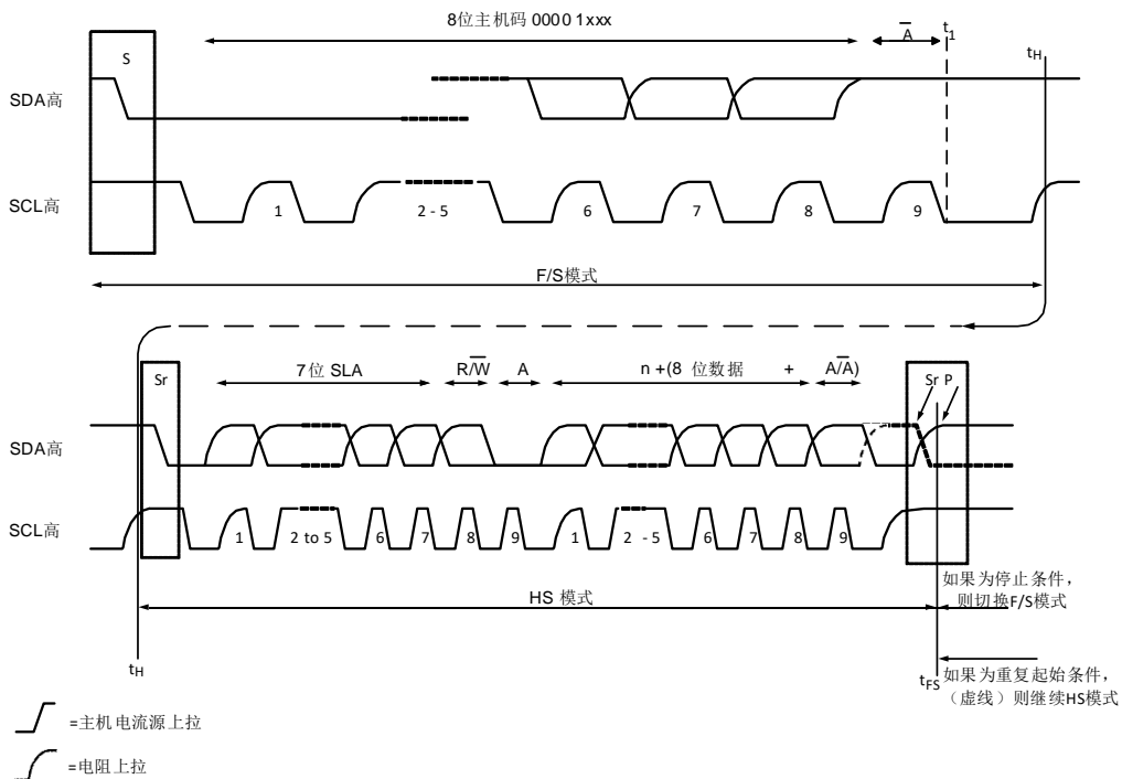
图 25 I 2 C 总线 HS 模式协议转换
