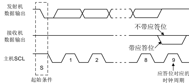
图 21 I 2 C 总线应答位
