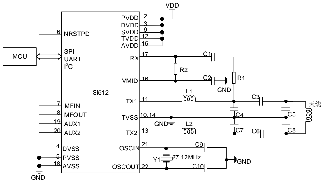
图 38 Si512 典型应用电路图-2
