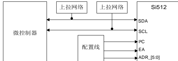
图 18 I 2 C 总线接口
