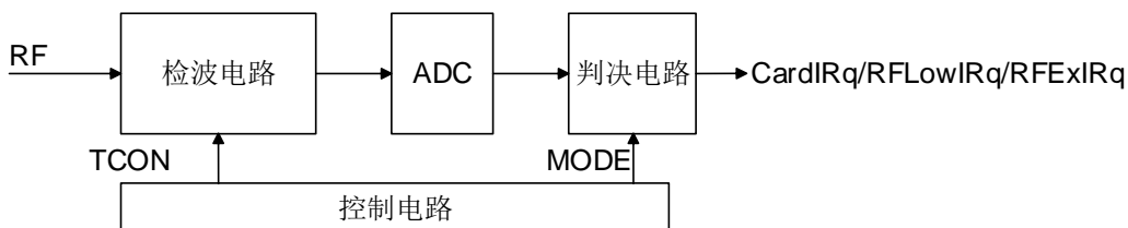
图 11 ACD 功能简图
