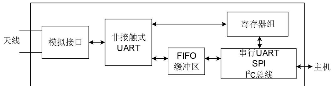
图 1 Si512 简化框图
