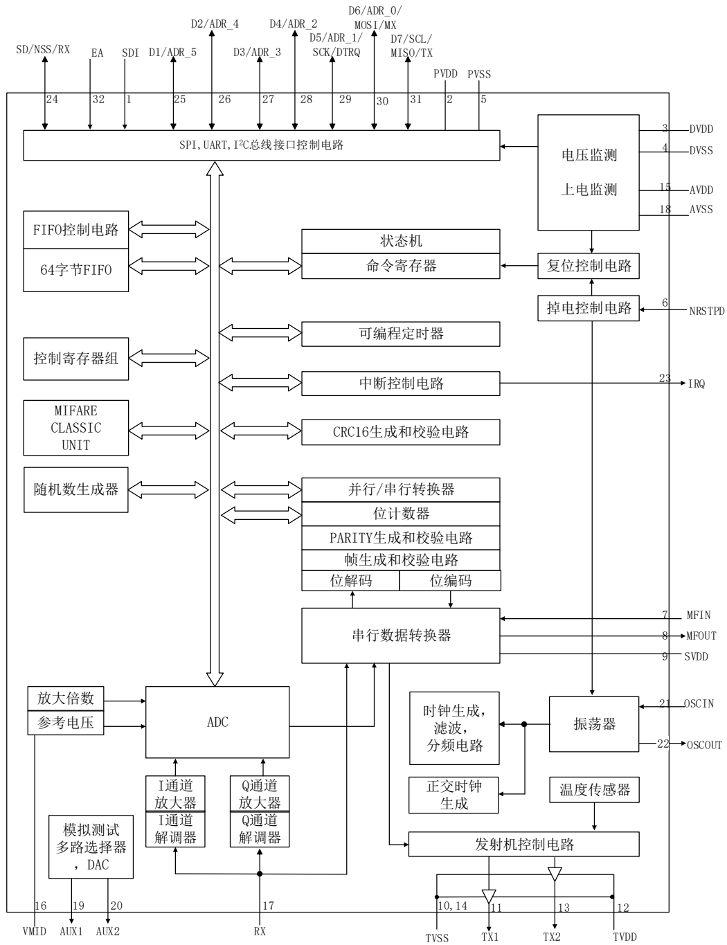
图 2 Si512 功能框图
