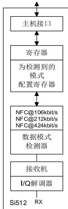
图 27 数据模式检测器
