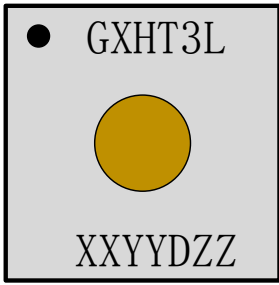
图 8 GXHT3L-DIS 顶视图以及激光标记
