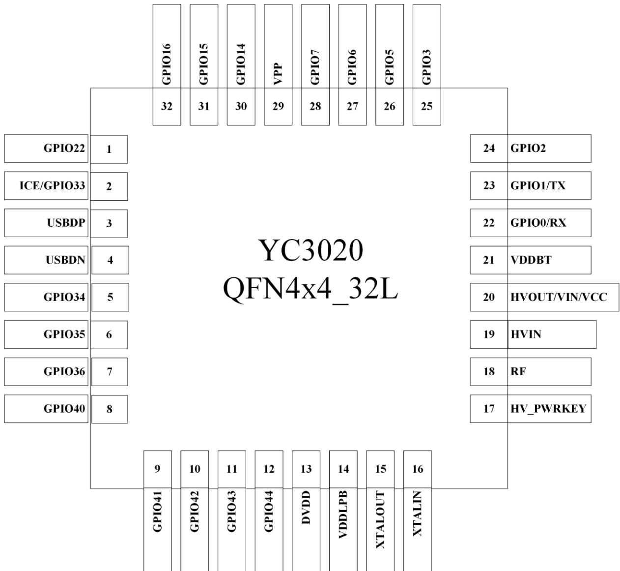
图 3 QFN32L 芯片管脚图
