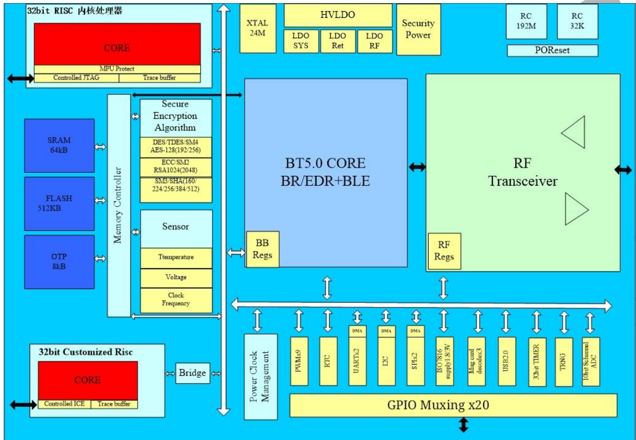
图 1 系统架构图
