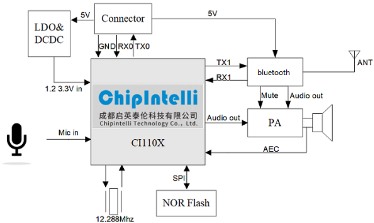
图1 模块框图
