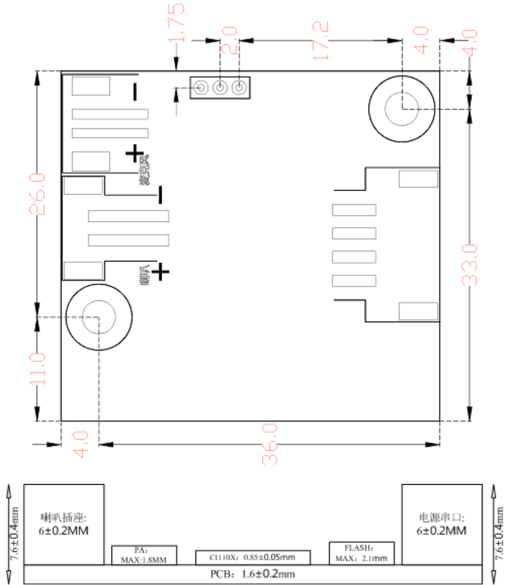
图5 模块尺寸图
