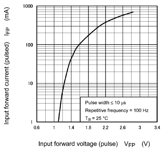
Fig. 11.6 I_{FP} - V_{FP}
