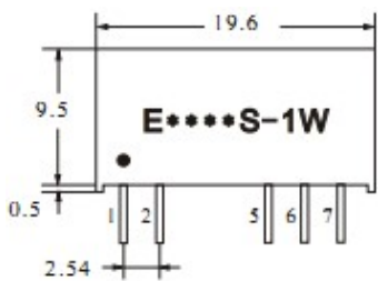
正视图
