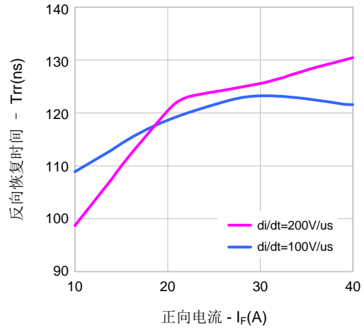
图16. 反向恢复时间vs正向电流
