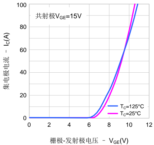
图4. 传输特性
