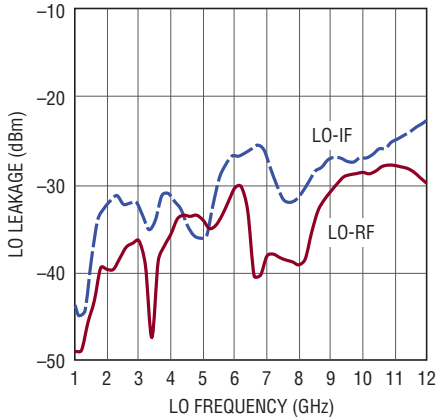
LO Leakage
