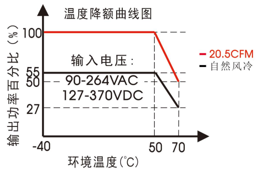
LOF350-20B15(满载 325W 带 20.5CFM 风扇)
