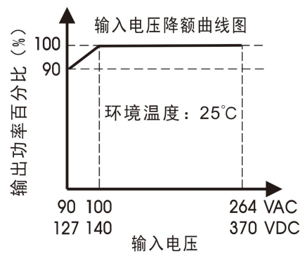
LOF350-20Bxx 输入电压降额
