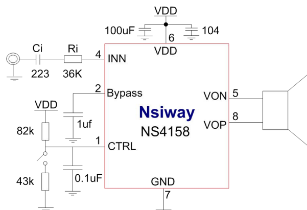
图 1 NS4158 典型应用电路
