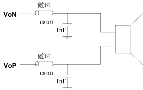
图 11 输出端加磁珠应用图
