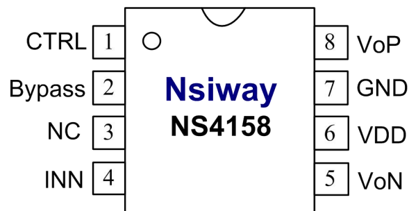
图 2 NS4158 封装管脚分配图(top view)
