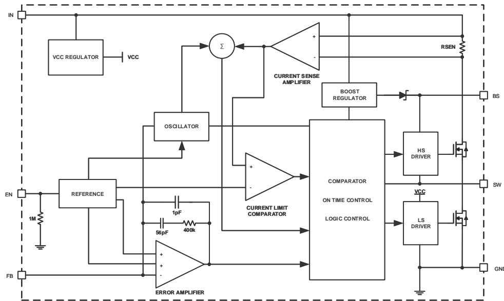
Figure 2. RY8134A Block Diagram
