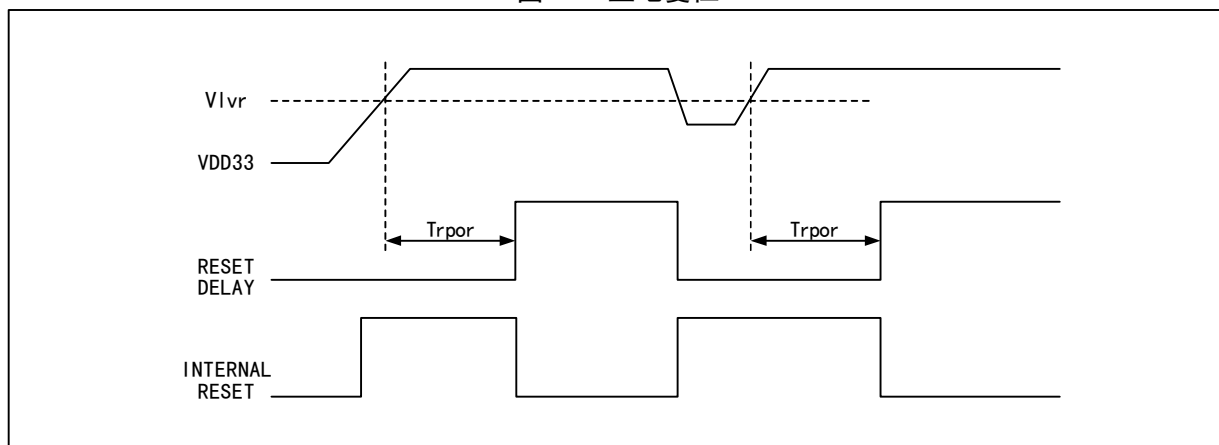
图 3-1 上电复位
