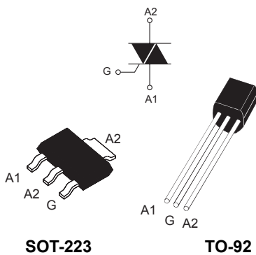
SOT-223
