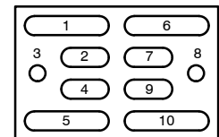
WLCSP10 (3.20 x 2.10 x 0.14) CASE 567XT
