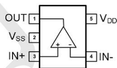
SOT23-5
