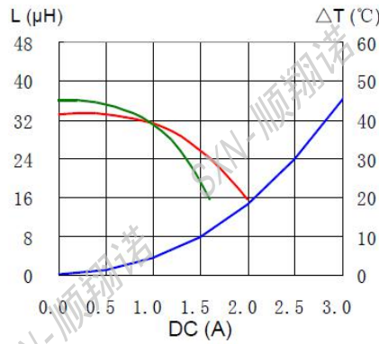
SMRH8D58-330N
