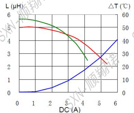
SMRH8D58-5R0N
