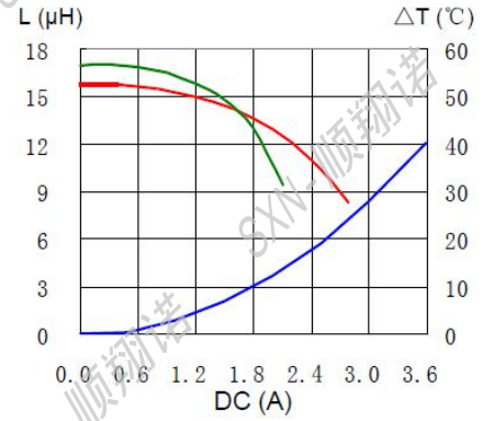
SMRH8D58-150N
