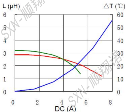
SMRH8D58-2R8N
