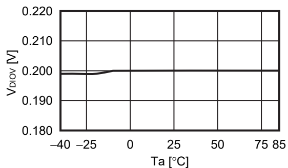
2.7 V_{DIOV} - T_a
