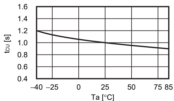
2.5 t_{CU} - T_a
