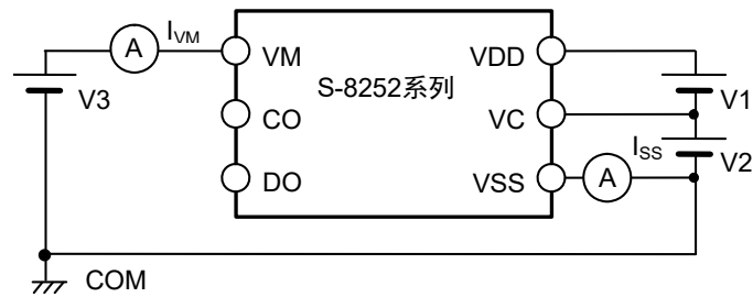
图7 测定电路3
