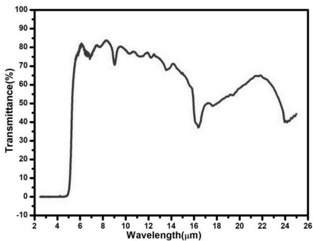
图 4. 滤光片的透过光谱
