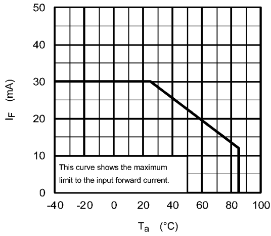
Fig. 16.1.1 I_F - T_a
