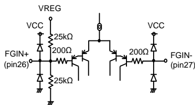
○ OFG amplifier input
