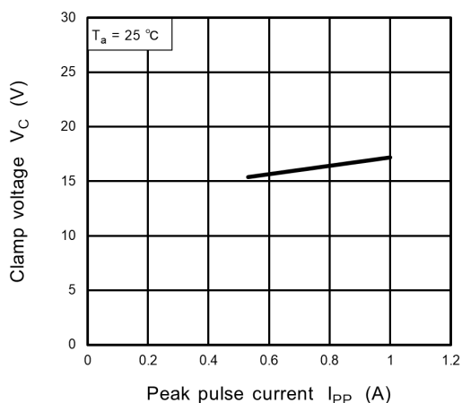
Fig. 6.2.1 V_C - I_{PP}
