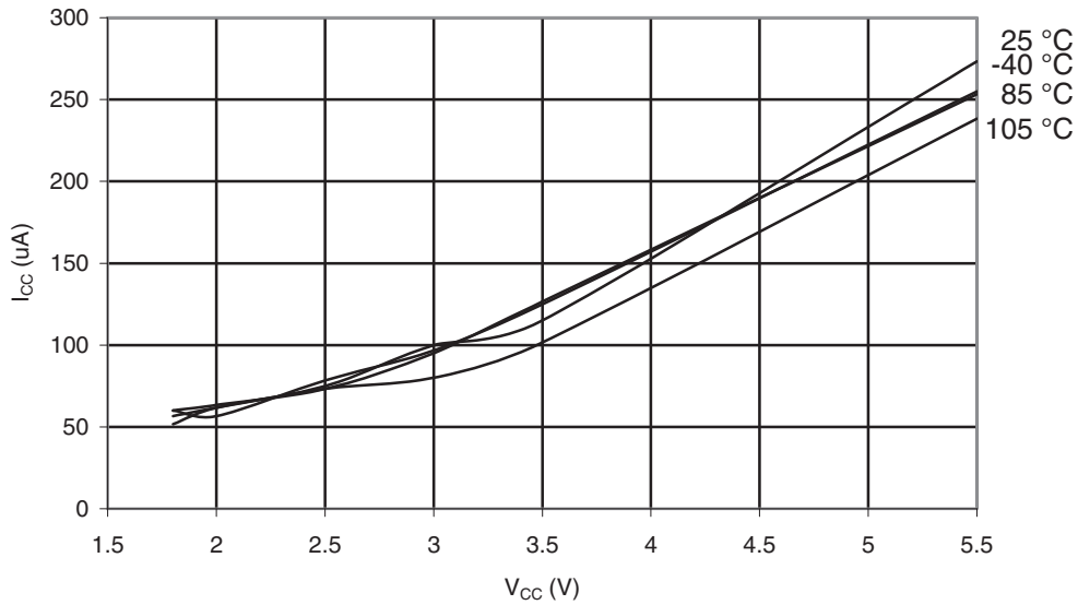
Figure 31-74. ADC Current vs. V CC (AREF = AV CC )
