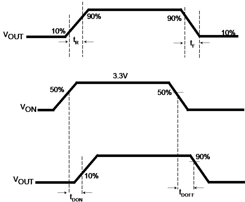
图 7. FPF1504时序图
