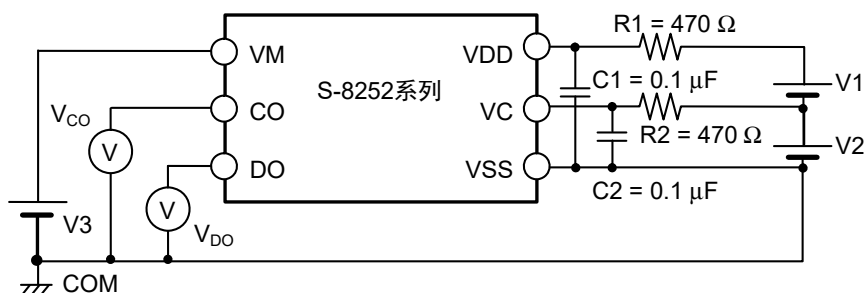
图5 测定电路1
