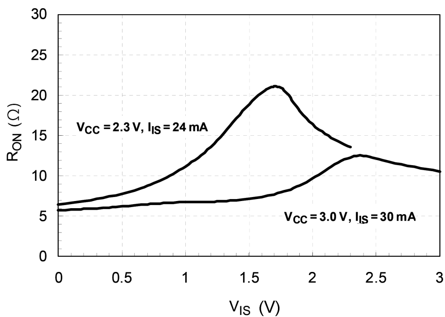
Fig. 13.1 R_{ON} - V_{IS} ( T_a = 25\text{ }^\circ\text{C} )
