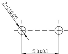
P.C.B LAND DIMENSION
