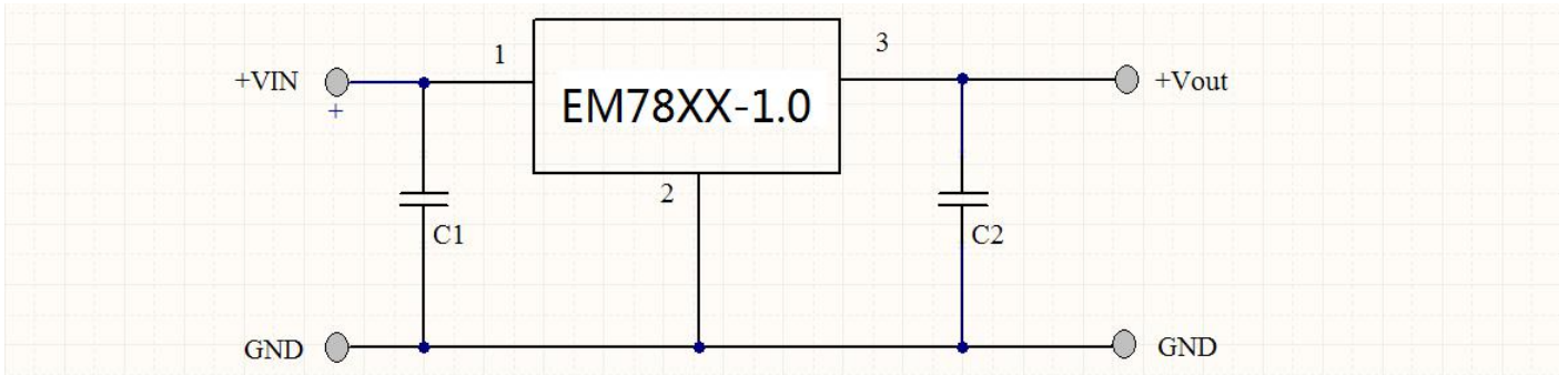
图 6：典型应用电路图
