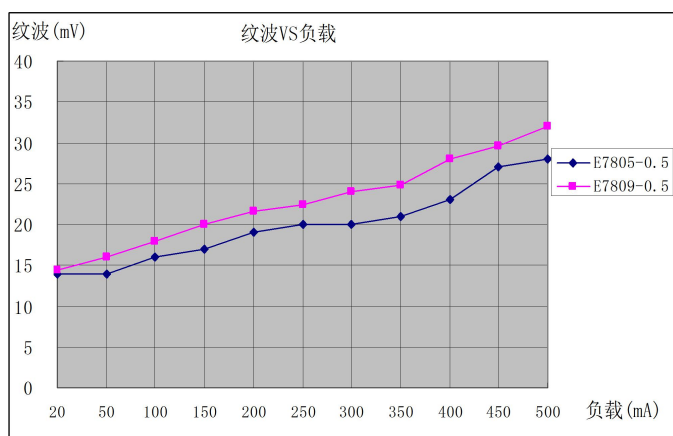
图 4: 纹波 VS 负载
