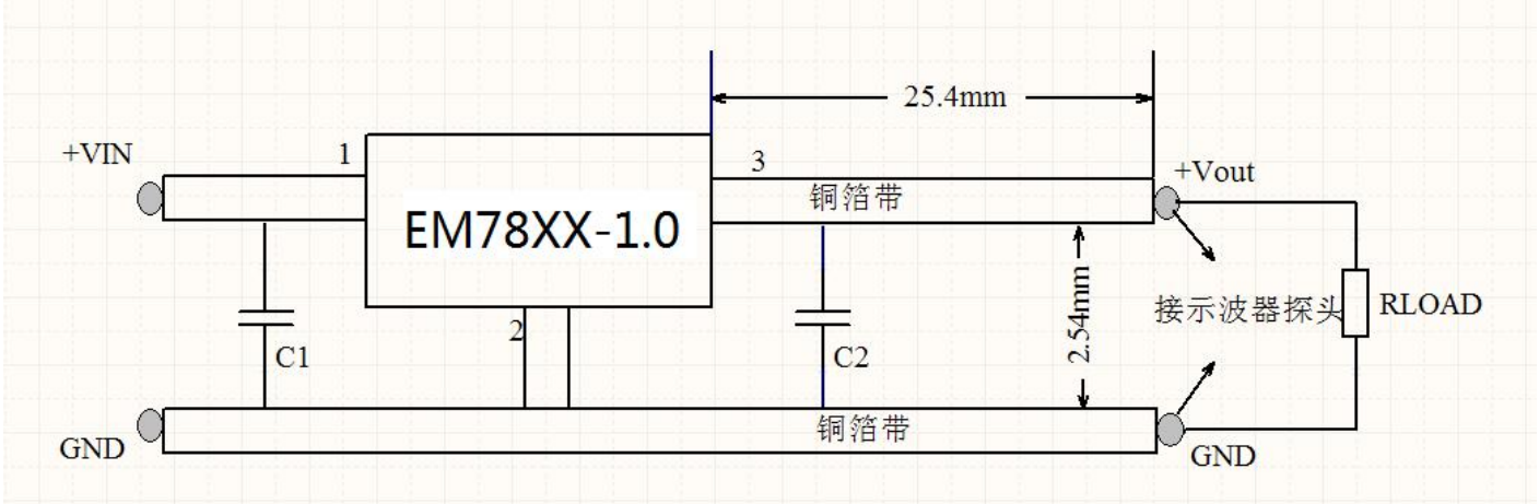
图 9：动态负载测试推荐图
