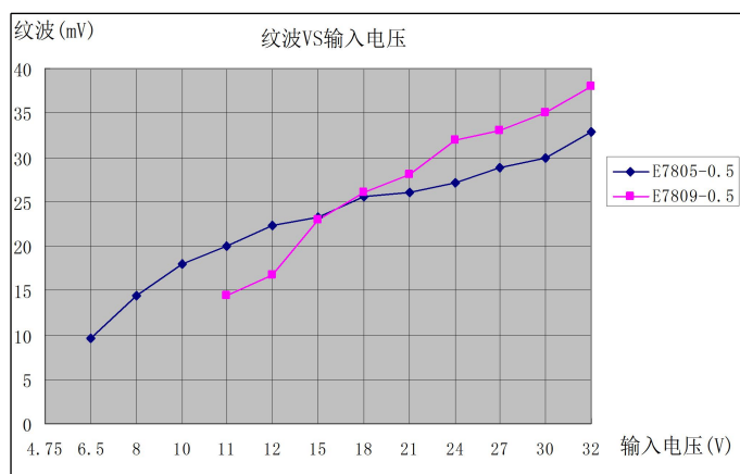
图 3: 纹波 VS 输入电压
