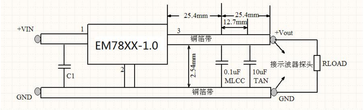
图 8：平行线测试法
