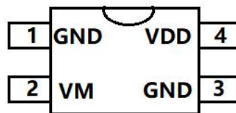
TSOT23-4
