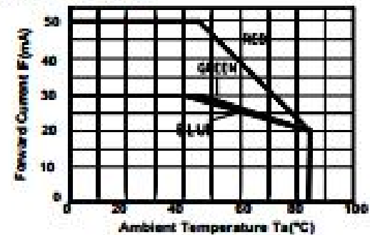
8). Thermal Design
