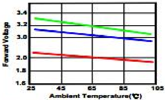
8). Thermal Design
