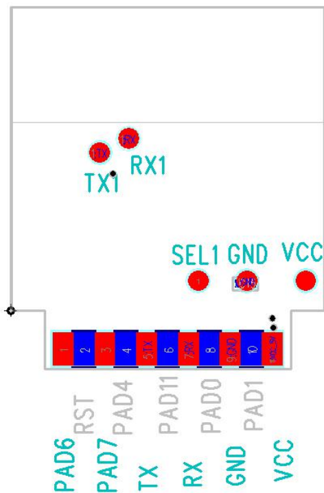
图3 引脚分布正视图
