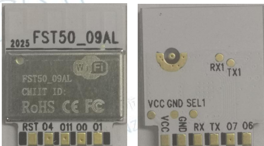
图 1 FST50_09AL 模组
