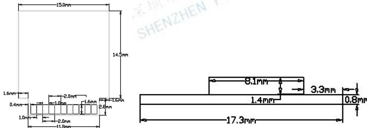
图 5 FST50_09AL 模组尺寸平面图 (单位: mm)
