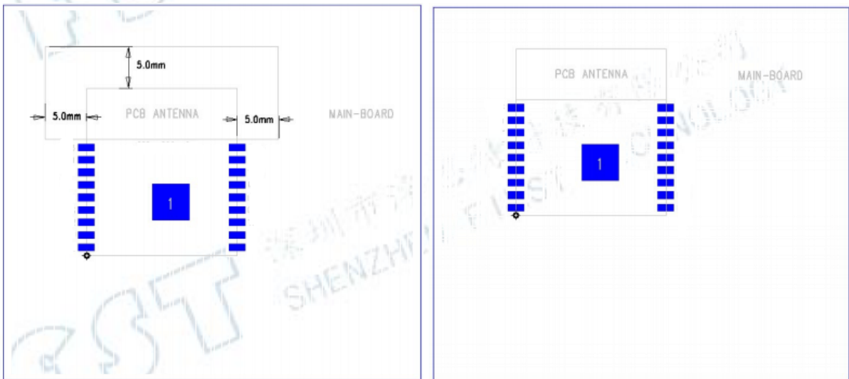
↑方案5：天线板框内放置且下方挖空
