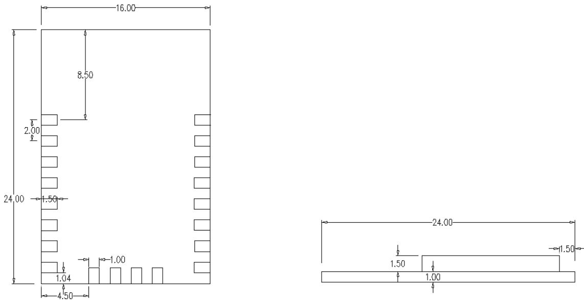
图 5 FST50_04EL 模组尺寸平面图（单位：mm）
