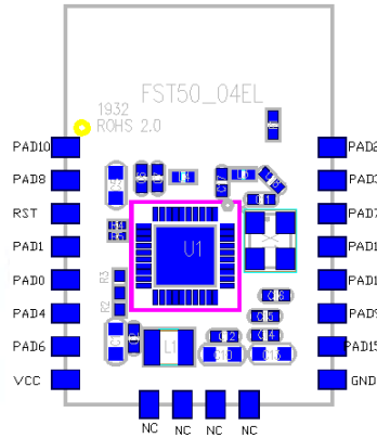
图 3 引脚分布正视图
