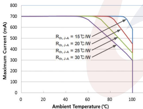
降额曲线
