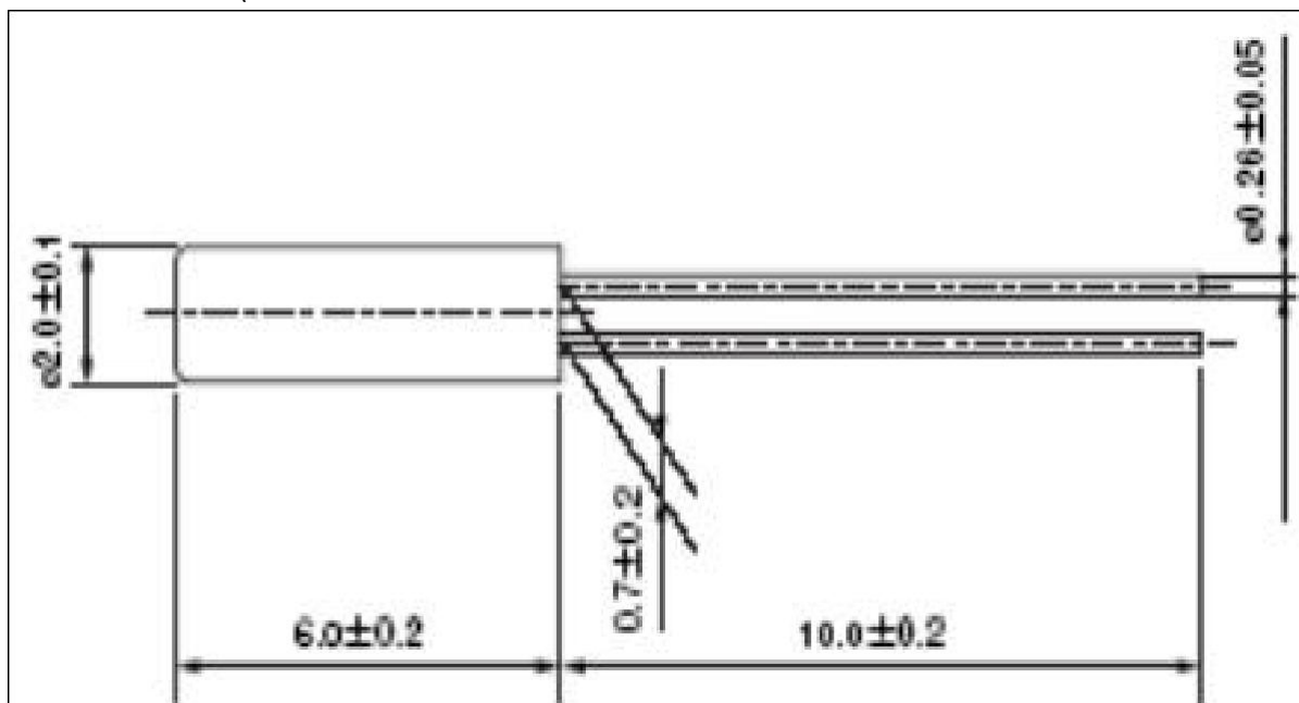
OUTLINE DIMENSIONS(UNIT:mm) 外形尺寸 (单位: mm)
