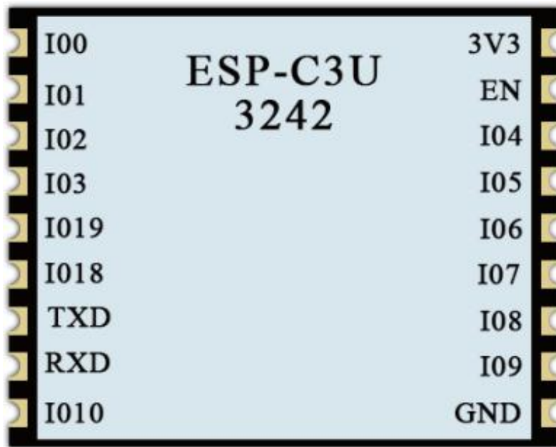
ESP32-C3U 管脚示意图
