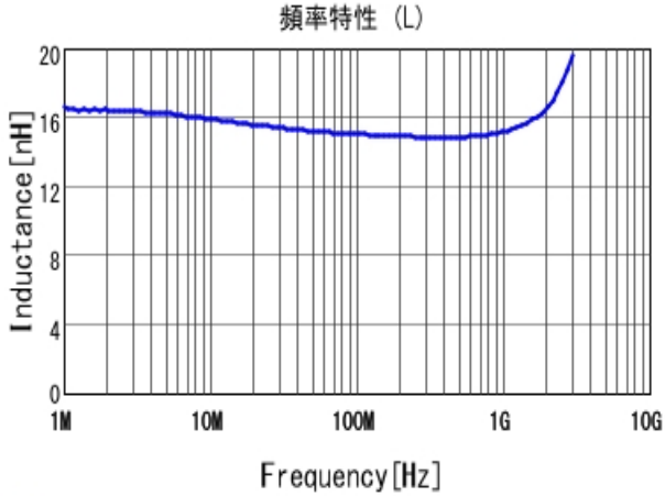
■ LQW18AN15NG80 L
