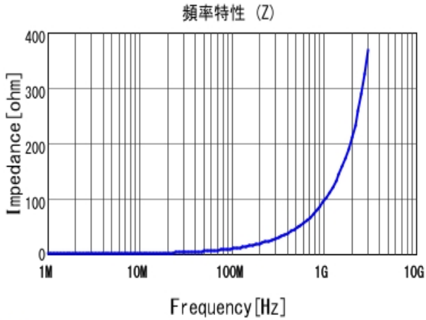
■ LQW18AN15NG80 |Z|
