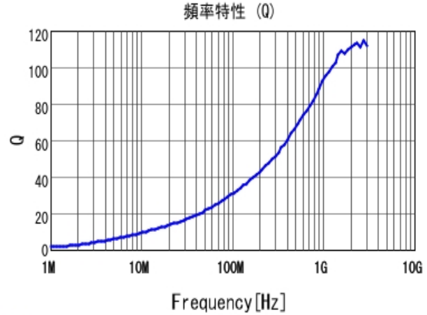
■ LQW18AN15NG80 Q
