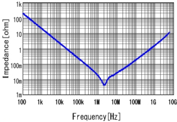
■ GRM188C80J106MEA6 |Z| DCOV, 25degC
