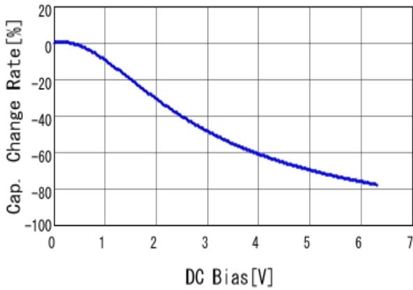
■ GRM188C80J106MEA6 C-DC bias capchange, 25.0degC, AC0.
