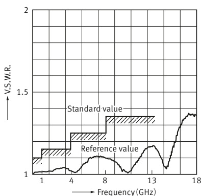
V.S.W.R.
