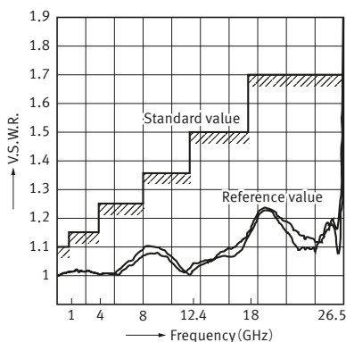
V.S.W.R.
