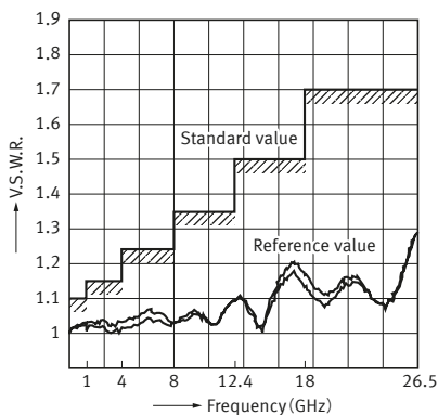
V.S.W.R.
