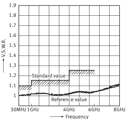
V.S.W.R.
