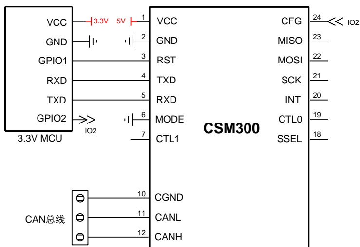
图 2.6 UART 转 CAN 参考电路 (CSM300)
