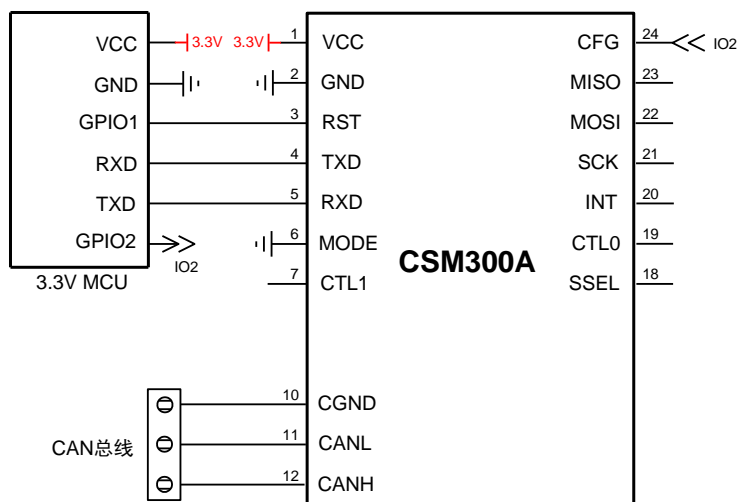
图 2.5 UART 转 CAN 参考电路 (CSM300A)
