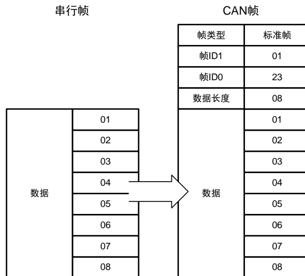
图 3.11 串行帧转 CAN 帧示例 1（透明转换）
