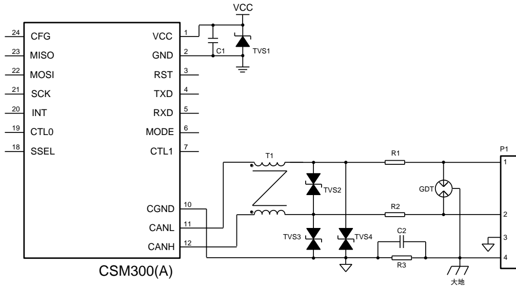
图 2.7 外围保护电路 1
