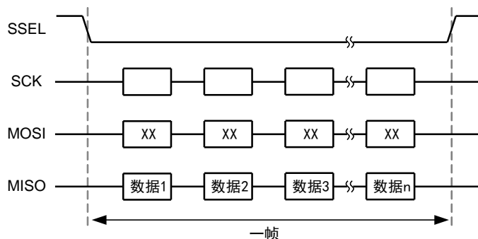
图 3.3 主机读数据帧示意
