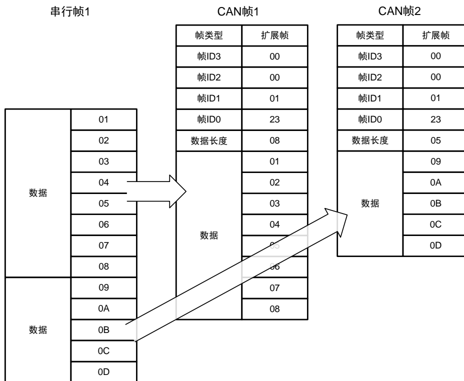
图 3.12 串行帧转 CAN 帧示例 2 (透明转换)
