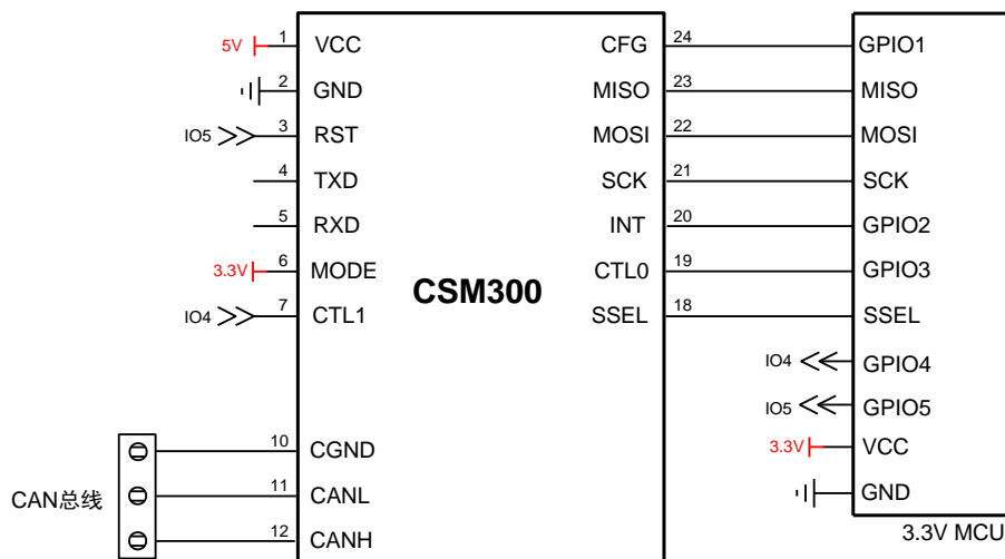
图 2.4 SPI 转 CAN 参考电路 (CSM300)
