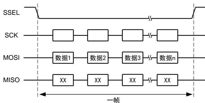
图 3.4 主机写数据帧示意
