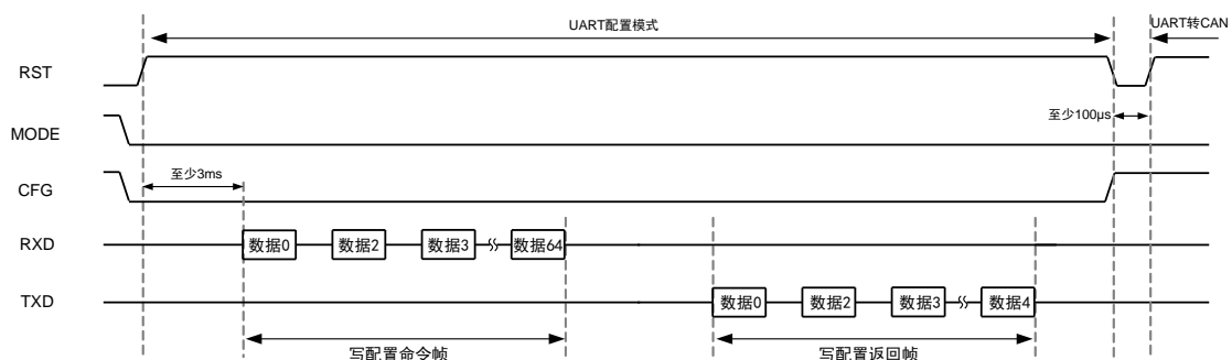
图 4.2 通过 UART 写配置命令时序图
