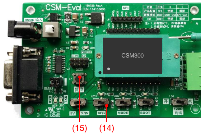
图 5.7 步骤 (14) ~ (15) 示意图
