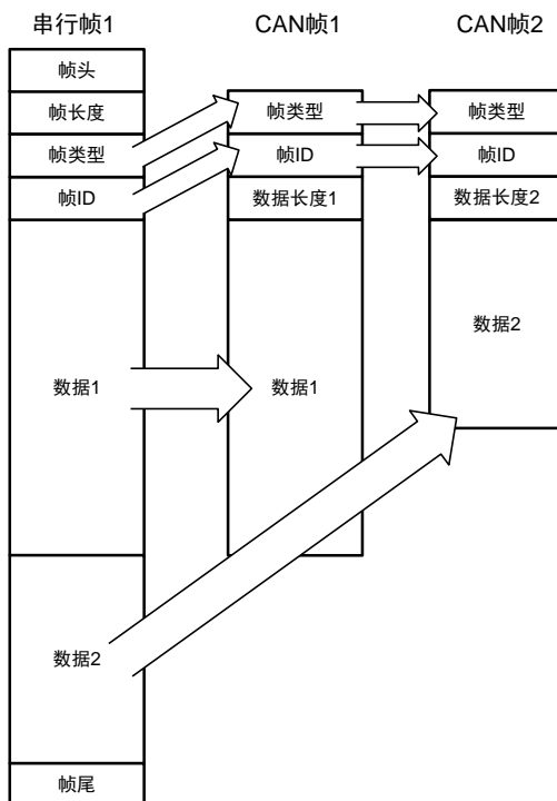
图 3.29 串行帧转 CAN 帧 2 (自定义协议转换)
