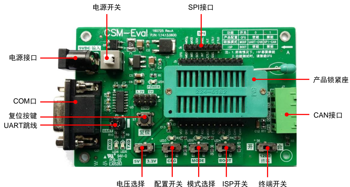
图 5.2 CSM-Eval 评估板
