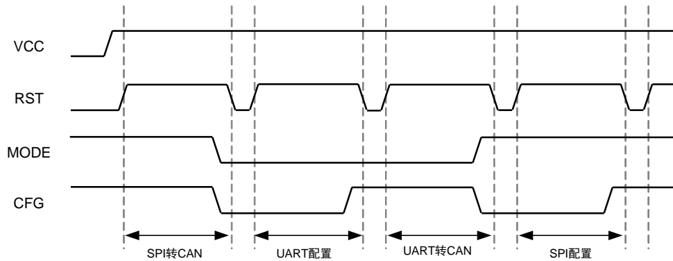
图 3.2 工作模式切换时序
