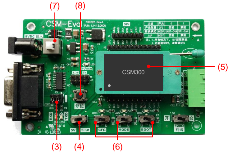
图 5.4 步骤（2）~（8）示意图
