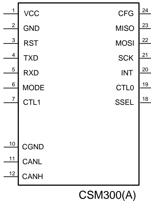
图 2.2 引脚排列
