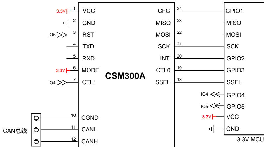
图 2.3 SPI 转 CAN 参考电路 (CSM300A)
