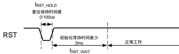
图 3.1 复位时序示意图
