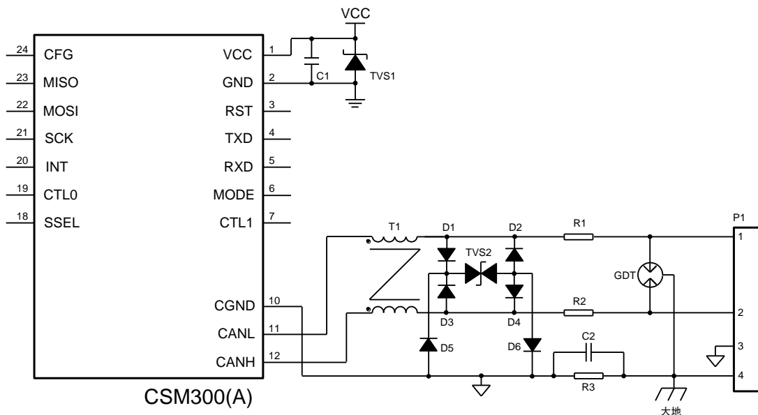
图 2.8 外围保护电路 2
