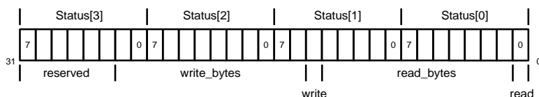
图 3.6 状态字节数据结构
