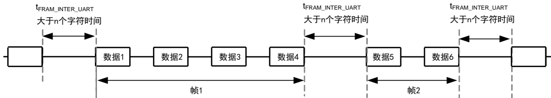
图 3.8 UART 通信帧格式
