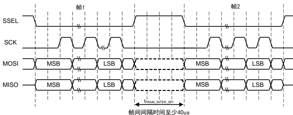
图 3.5 SPI 帧间隔示意图
