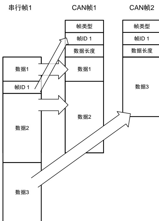
图 3.22 串行帧转 CAN 帧（透明带标识转换，数据大于 8 个字节）
