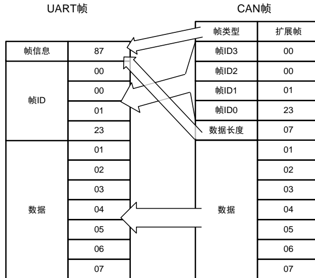
图 3.16 CAN 帧转 UART 帧示例（透明转换，帧信息、帧 ID 转换使能）
