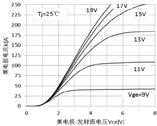
图 1 常温输出特性
