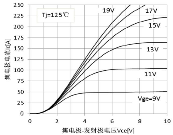
图 2 高温输出特性
