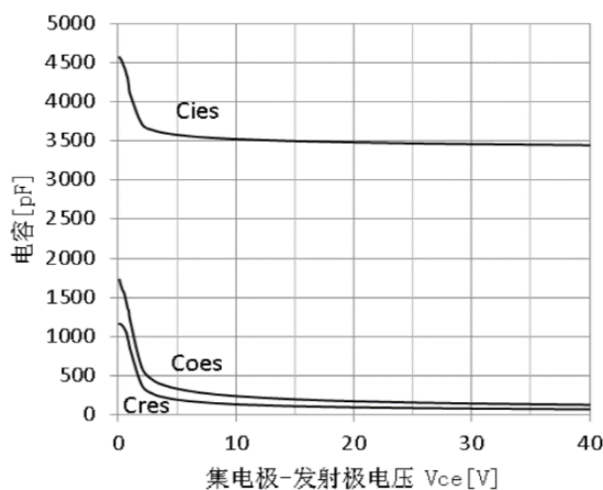
图 5 电容特性
