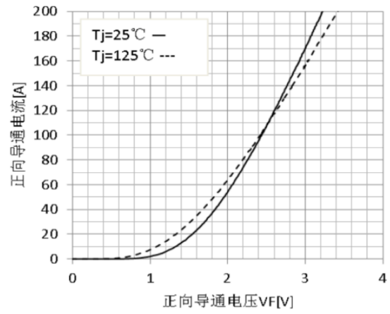
图 8 二极管正向特性
