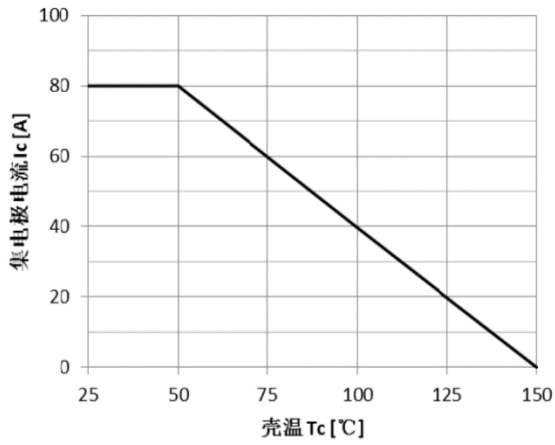
图 7 集电极电流温度特性
