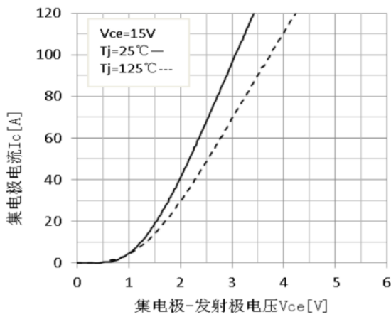
图 3 典型饱和和压降特性
