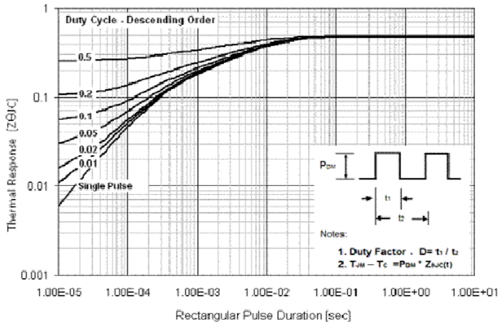
图 9 瞬态热阻特性
