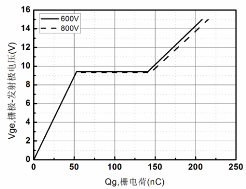
图 6 栅电荷特性
