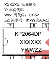
DIP-7
