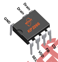
DIP-7
