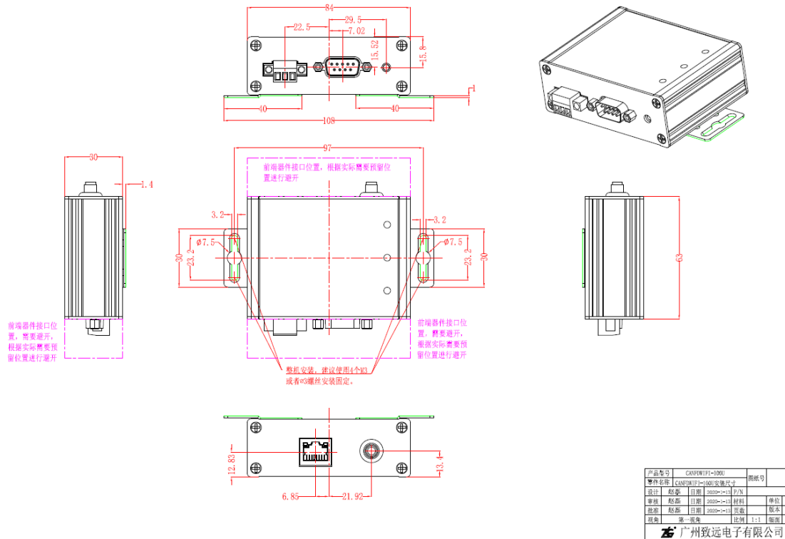
图 3.1 主机尺寸图
