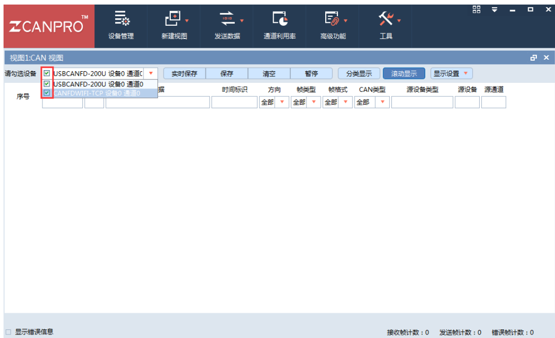
图 5.15 主界面视图
