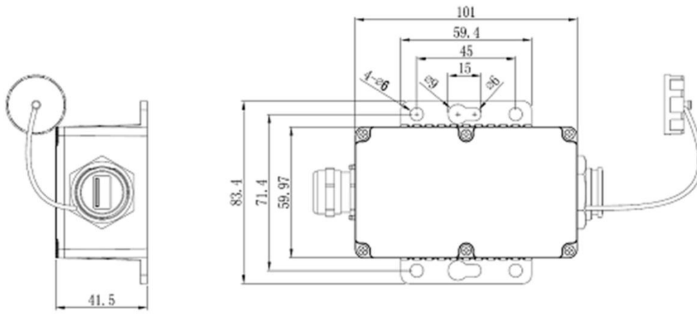
图 2.1 机械尺寸
