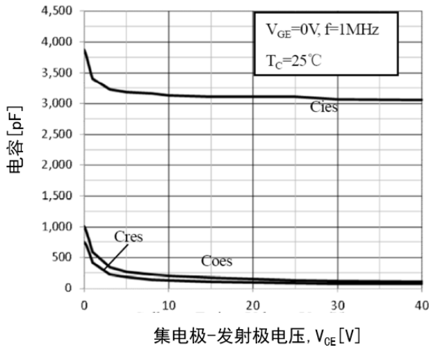
图 9 电容特性
