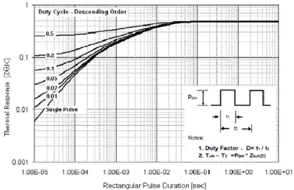
图 15 瞬态热阻特性
