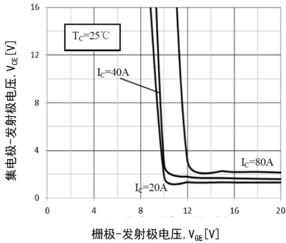
图 7 V_{CE(sat)}-V_{GE} 关系(常温)
