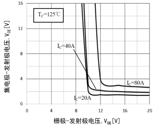
图 8 V_{CE(sat)}-V_{GE} 关系(高温)
