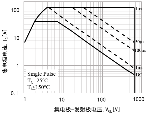
图 1 正偏安全工作区
