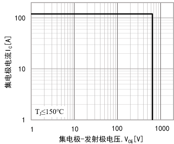
图 2 反偏安全工作区
