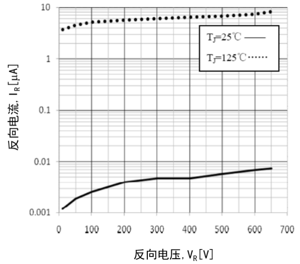
图 14 二极管反向特性
