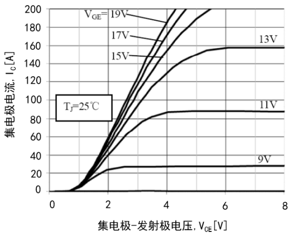
图 3 常温输出特性
