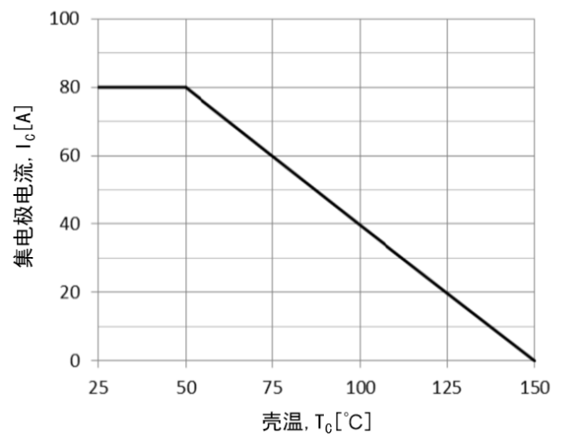
图 12 集电极电流温度特性
