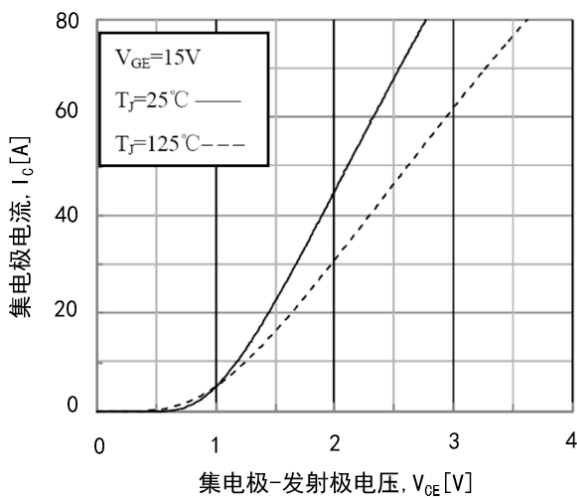
图 5 典型饱和压降特性
