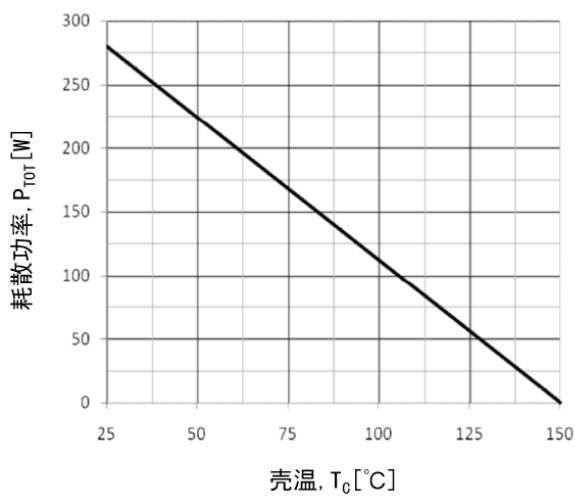
图 11 耗散功率-壳温关系
