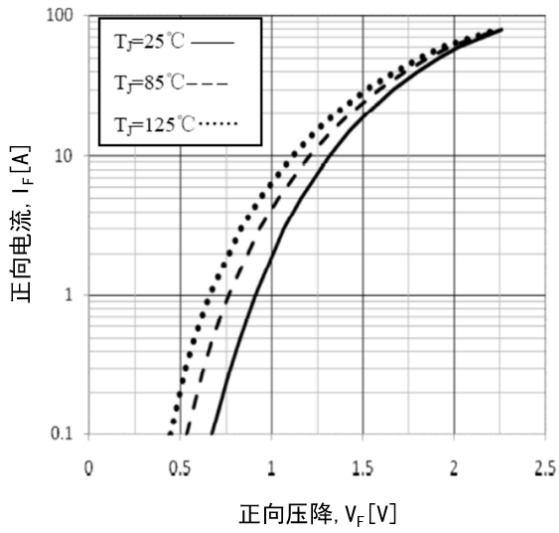
图 13 二极管正向特性
