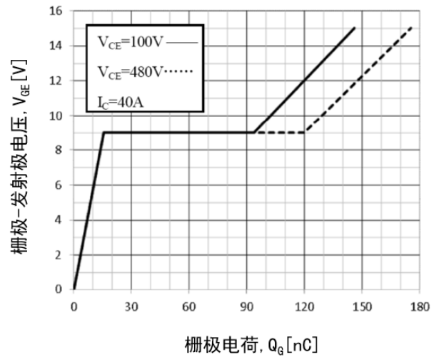
图 10 栅极电荷特性
