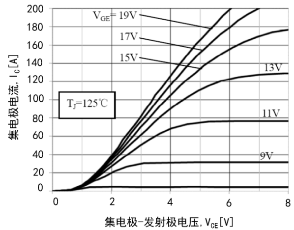
图 4 高温输出特性
