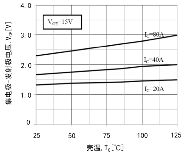
图 6 饱和压降温度特性
