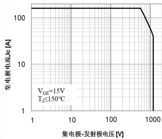
图 2 反偏安全工作区
