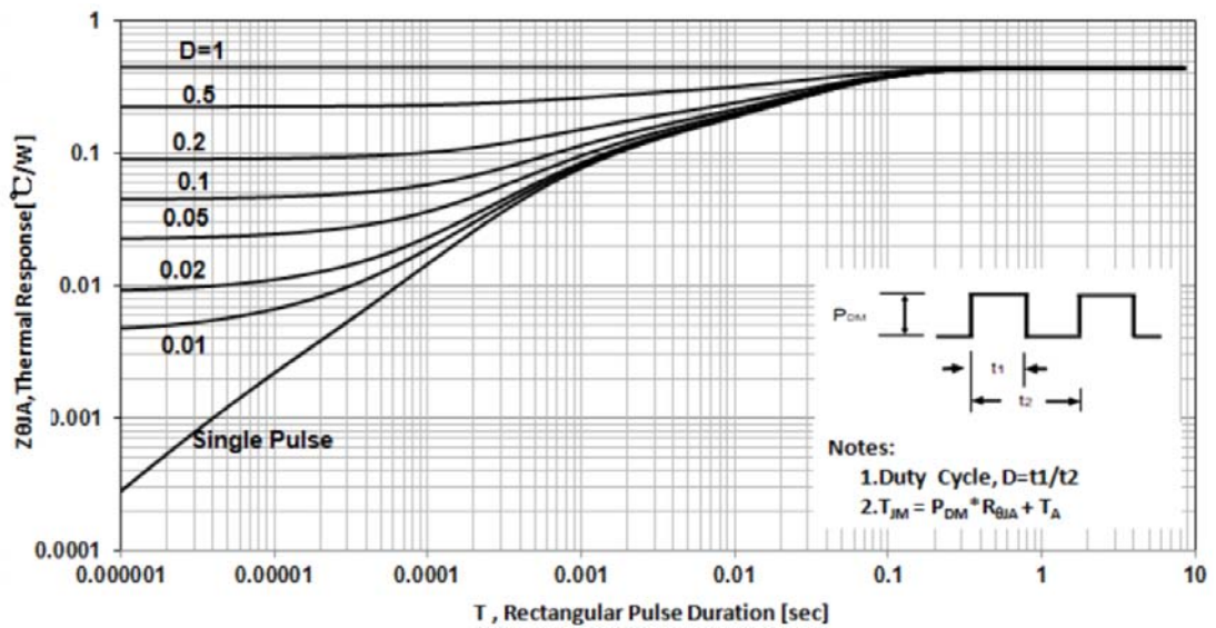
图 20 瞬态热阻特性
