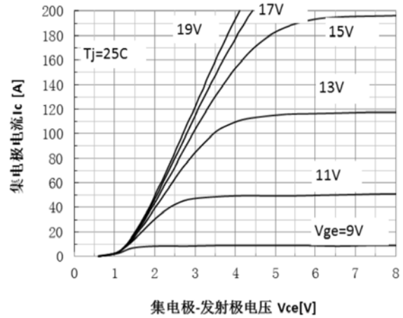
图 4 常温输出特性 (T j =25°C)
