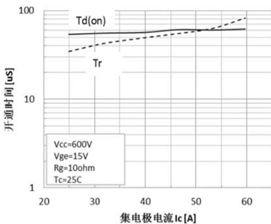
图 11 开通时间与集电极电流的关系
