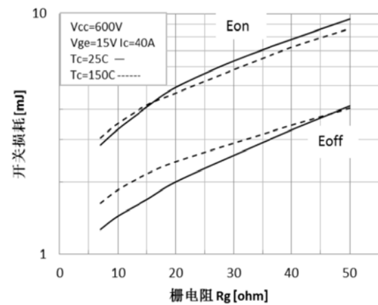
图 10 开关损耗与栅电阻的关系
