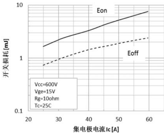
图 13 开关损耗与集电极电流的关系
