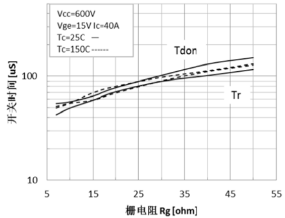
图 8 开通时间与栅电阻的关系
