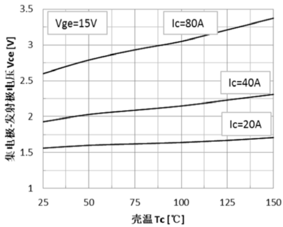
图 7 饱和压降温度特性
