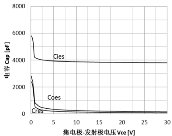
图 18 电容特性
