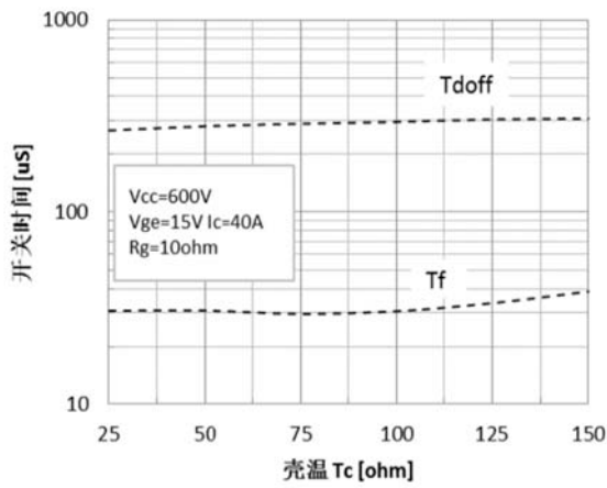
图 15 关断时间与壳温的关系
