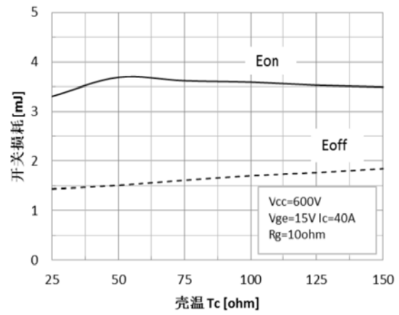
图 16 开关损耗与壳温的关系
