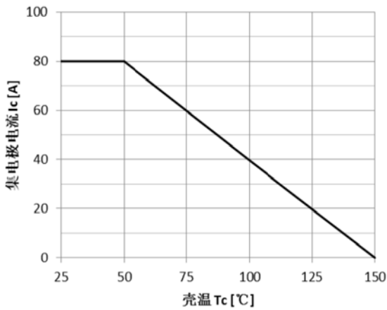
图 3 集电极电流温度特性
