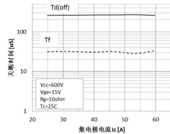
图 12 关断时间与集电极电流的关系
