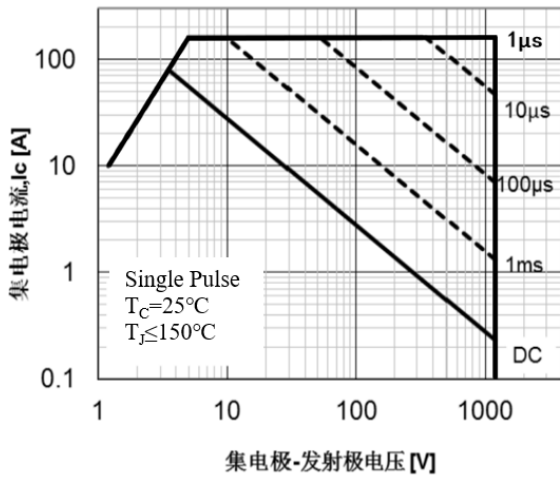
图 1 正偏安全工作区
