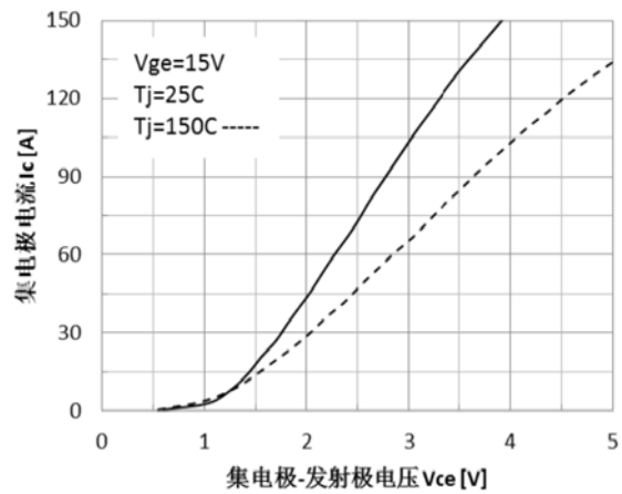
图 6 典型饱和和压降特性
