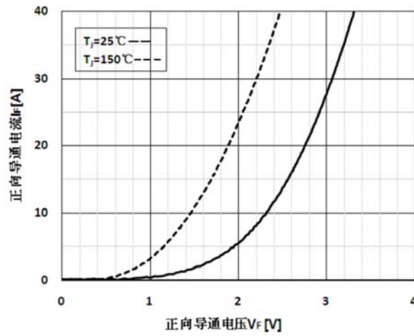
图 19 二极管正向特性
