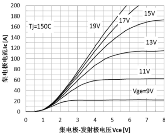
图 5 高温输出特性 (T j =150°C)
