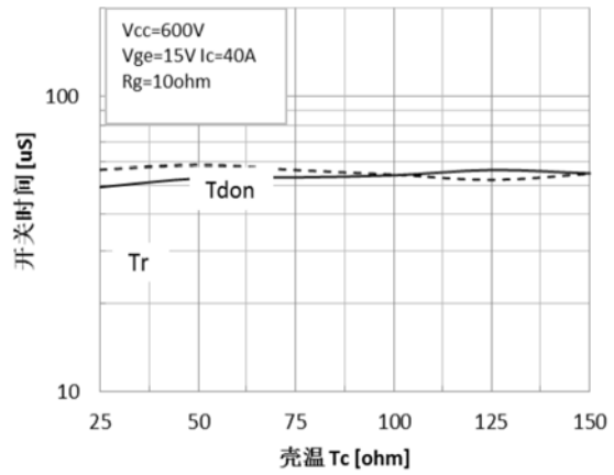
图 14 开通时间与壳温的关系
