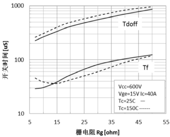
图 9 关断时间与栅电阻的关系
