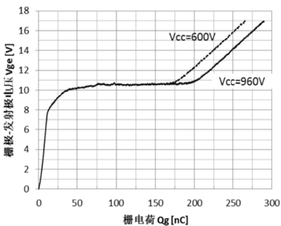
图 17 栅电荷特性
