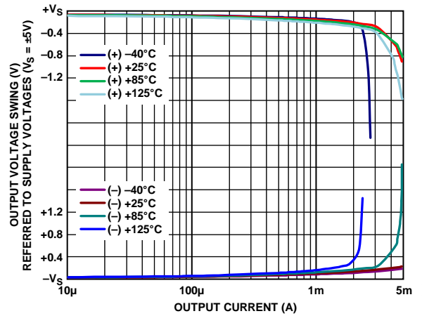
图25. 输出电压摆幅与输出电流的关系, V_s = \pm 5V
