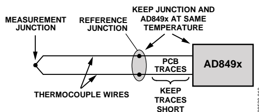
图31. 补偿热电偶基准结温
