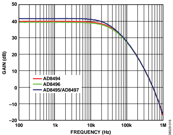
图5. 频率响应
