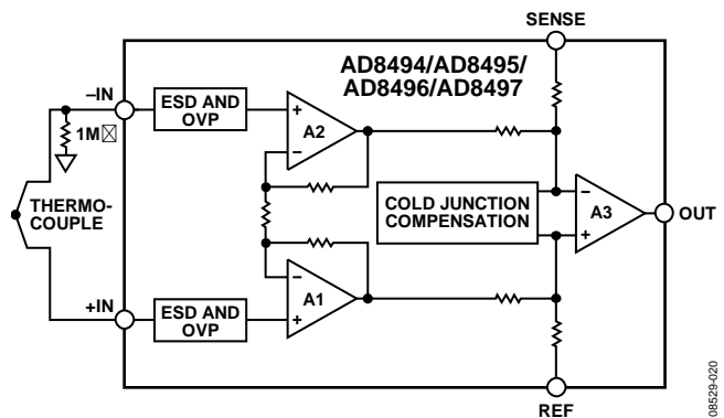
图27. 功能框图
