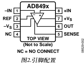
图2. 引脚配置
