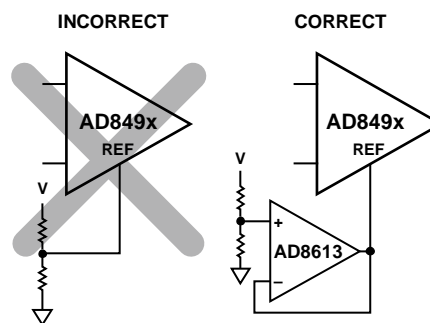
图32. 驱动基准引脚
